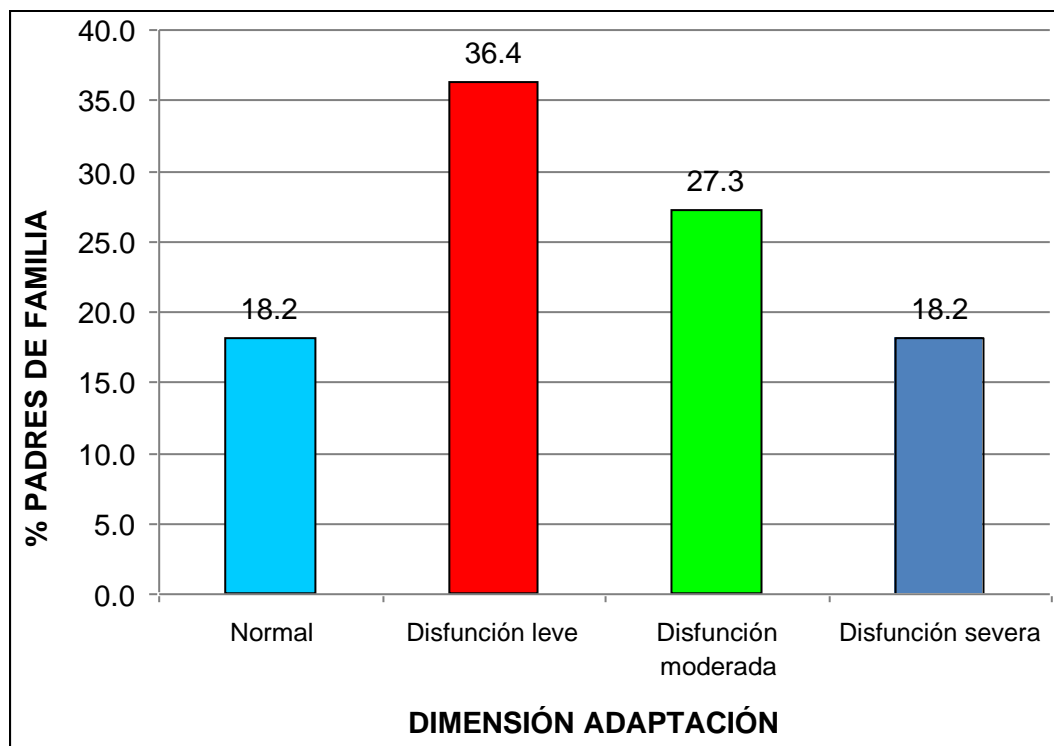
Gráfico 2. Dimensión adaptación
