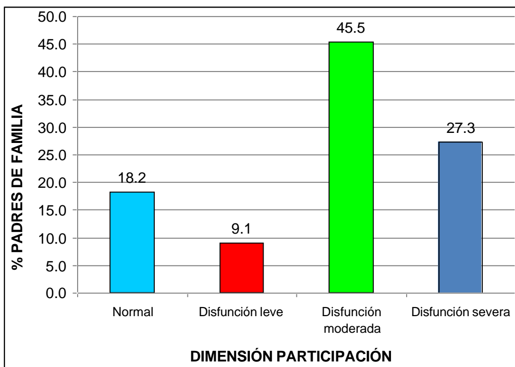
Gráfico 3. Dimensión participación
