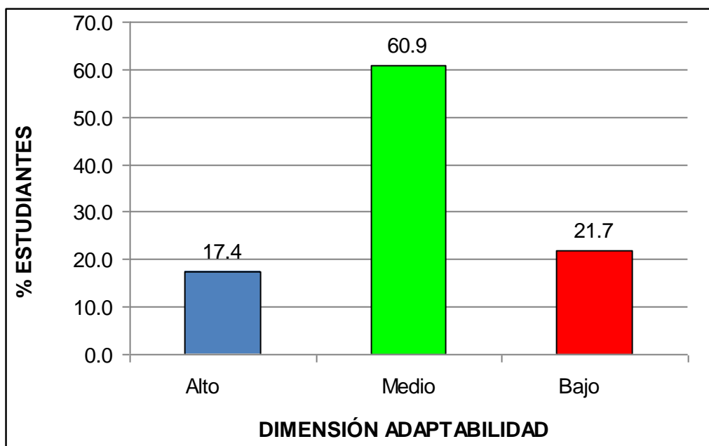
Gráfico 9. Dimensión adaptabilidad
