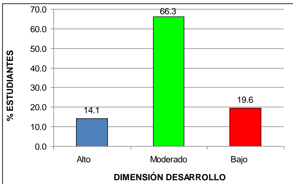
Gráfico 3. Dimensión desarrollo
