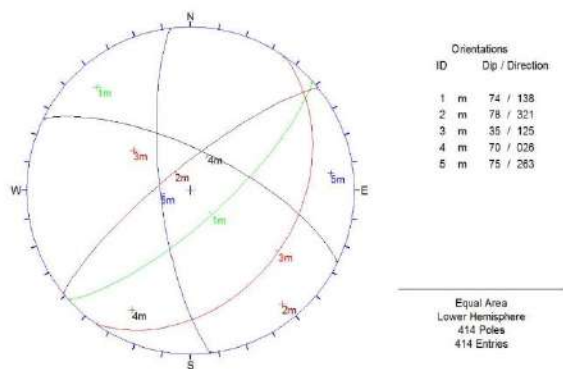
Figura 4.2: Diagrama estereográfico de planos principales del compuesto de discontinuidades.
